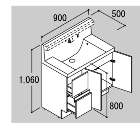
引出タイプ LCJ2HT-905SY/LD2H
